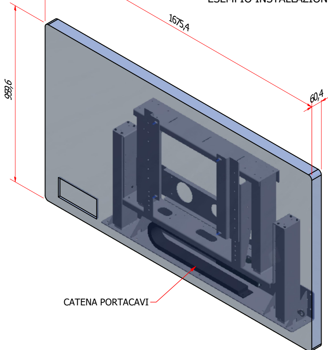
ESEMPIO INSTALLAZIONE TV 75"
